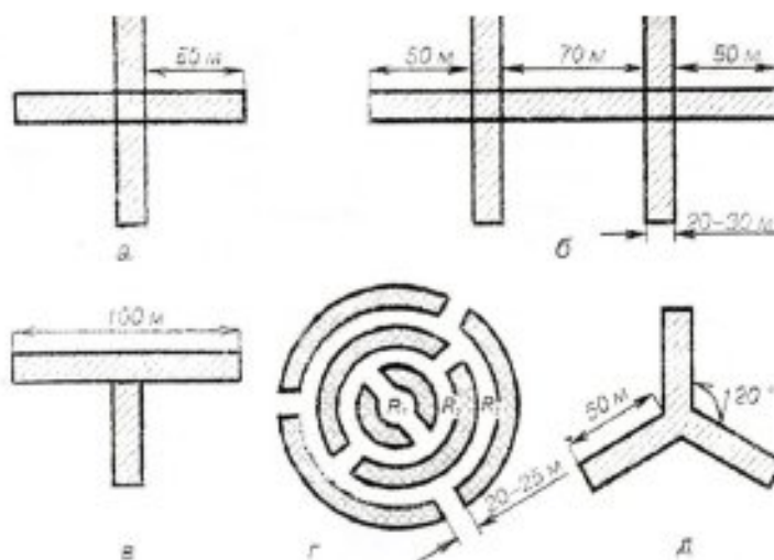
Рисунок 1 – Схема затишковых насаждений:
