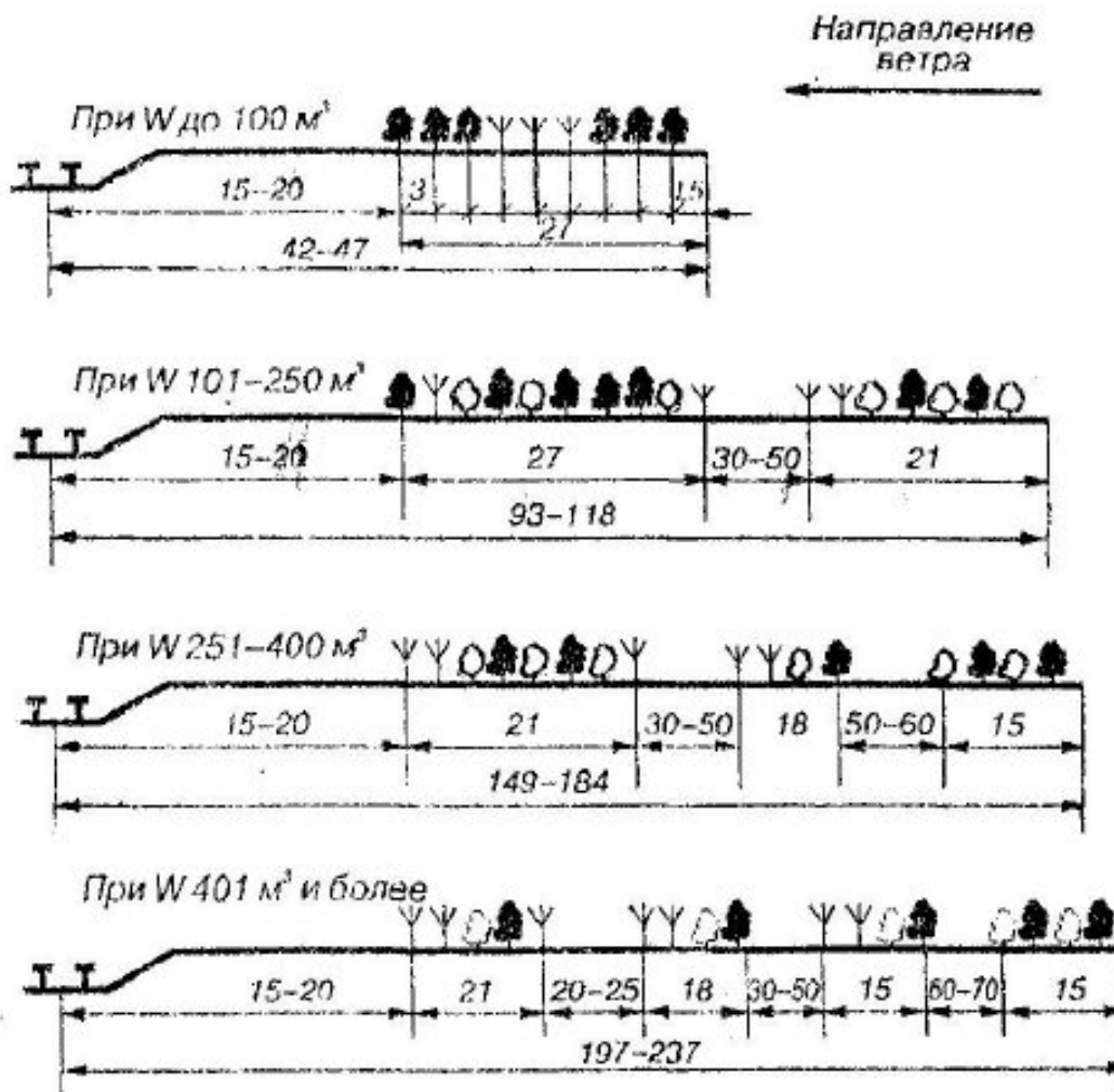
Рисунок 1 - Схемы снегозадерживающих лесных полос вдоль железных дорог
